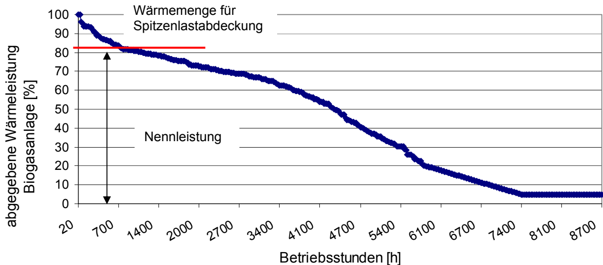
Abb. 5.: Beispiel für die Aufteilung zwischen Grundlast und Spitzenlast anhand einer Jahresdauerlinie der Heizleistung
