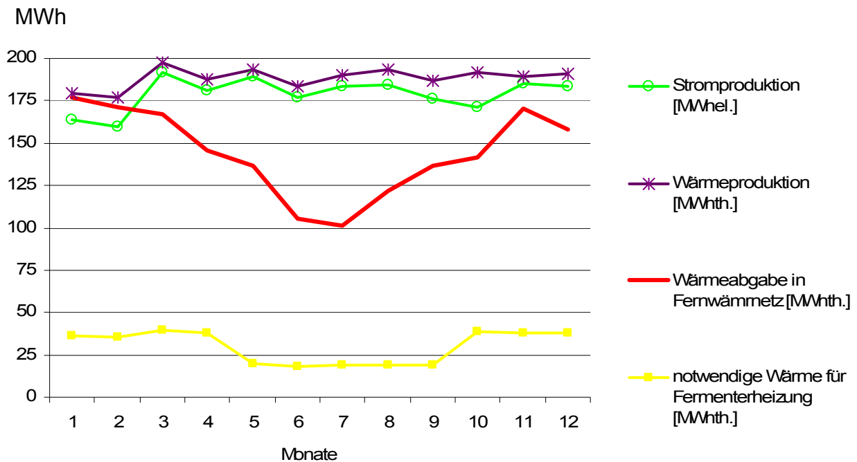
Abb. 4.: Sommer- und Winterlastgänge eines typischen Fernwärmernetzes mit einer Anschlussleistung von 250kW th.
