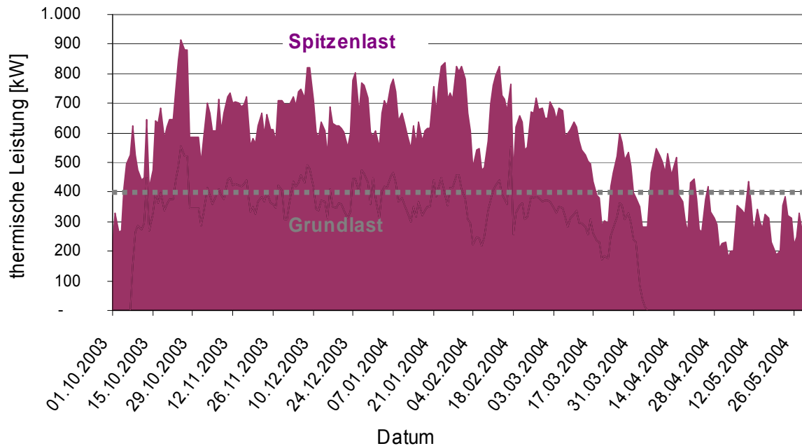
Abb. 10.: Praxisnahes Beispiel für eine Biogasanlage mit Spitzenlastproduktion
