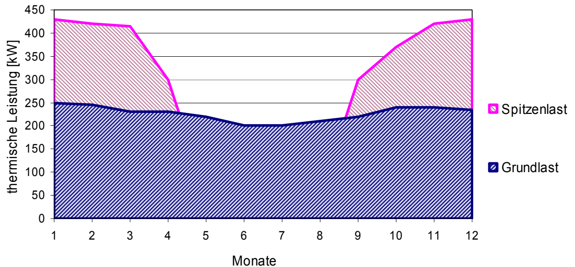
Abb. 9.: Nahwärme ohne garantierter Leistung
