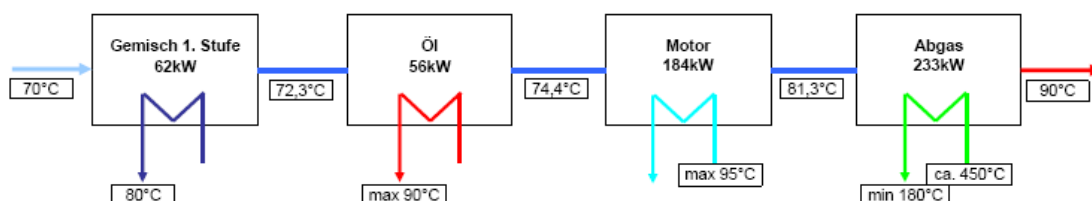
Abb. 1: Wärmequellen 500kW el BHKW, [GE JENBACHER]
